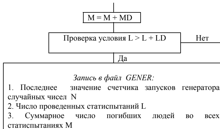
Рис 1. Структурная схема расчета Рнезв методом статиспытаний (Монте-Карло)
